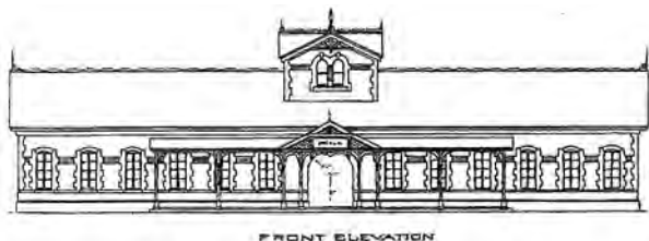
Figura 12. Fachada de vía, casa de estación Puebla del antiguo Ferrocarril Mexicano del Sur. Fuente: Mexican Southern Railway, Passenger Station Puebla (plano), México, 1890.
