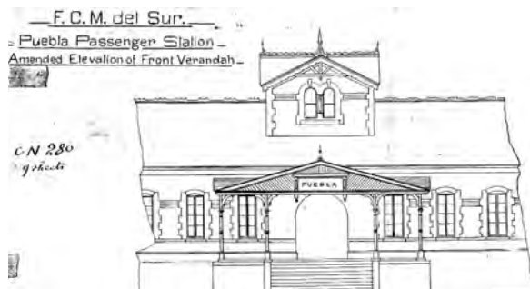
Figura 13. Fachada de la estación Puebla del antiguo Ferrocarril Mexicano del Sur. Fuente: idem.
